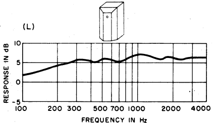
Fig. 3 - I dodici differenti tipi di cassa studiati da Olson e le relative curve di risposta. La cassa ideale sarebbe quella sferica (A) non considerando però la complessità costruttiva.
